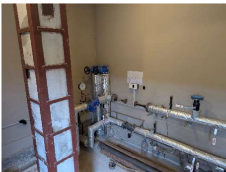
SKATS UZ VĒRTĒJAMĀ OBJEKTA – DAUDZDZĪVOKĻU DZĪVOJAMĀS MĀJAS JAUNBŪVES SILTUMMEZGLU
