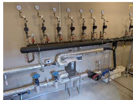
SKATS UZ VĒRTĒJAMĀ OBJEKTA – DAUDZDZĪVOKĻU DZĪVOJAMĀS MĀJAS JAUNBŪVES SILTUMMEZGLU
